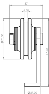
DÉTAIL GUIDE HAUT
