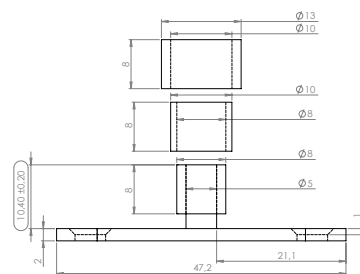
DÉTAIL GUIDE SOL
