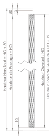
coupe verticale
